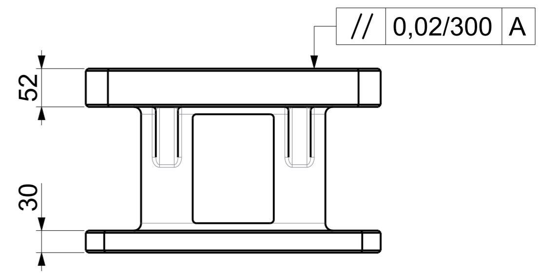
RISER TABLE - GIRD HOLE Art.No. FG/WH/RISTL/RTGRDNP004 Model.No. RTG/RT/800400/250-12
