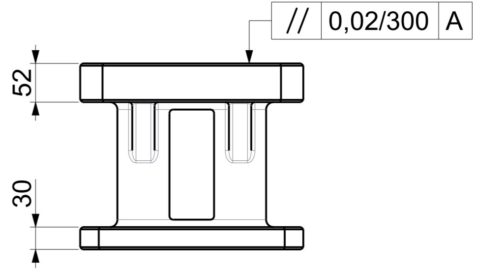
RISER TABLE - GIRD HOLE Art.No. FG/WH/RISTL/RTGRDNP003 Model.No. RTG/RT/600300/250-12
