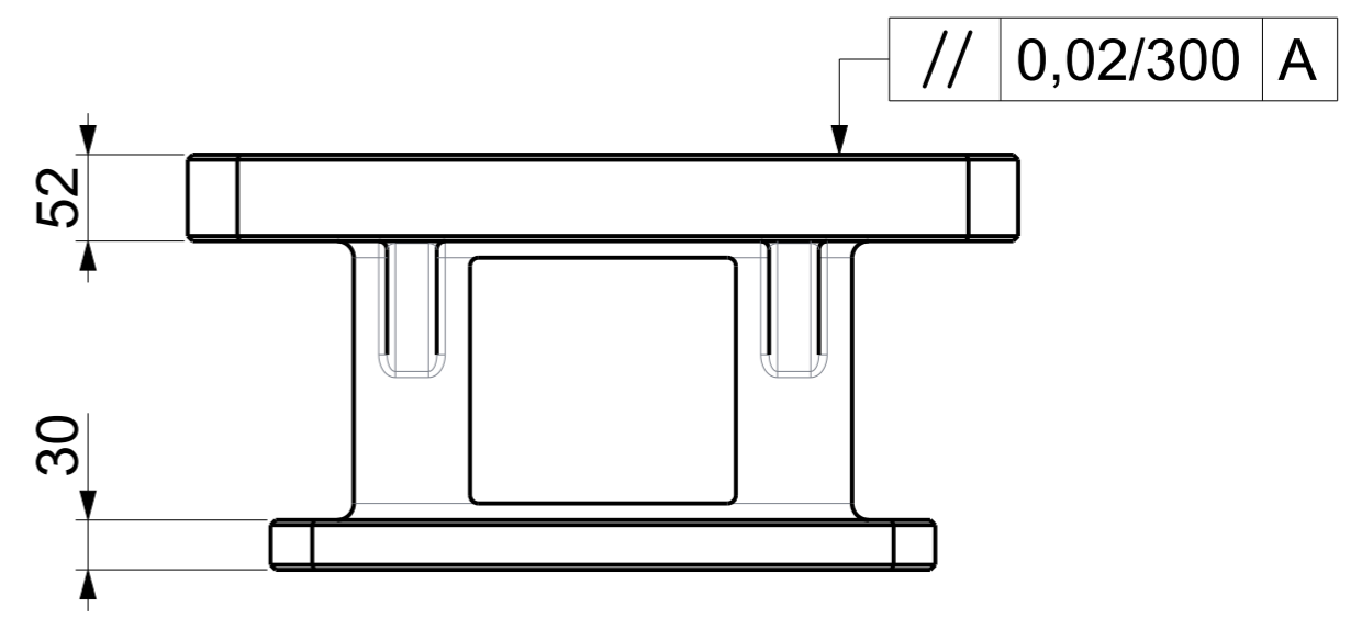
RISER TABLE - GIRD HOLE Art.No. FG/WH/RISTL/RTGRDNP002 Model.No. RTG/SQ/500500/250-12
