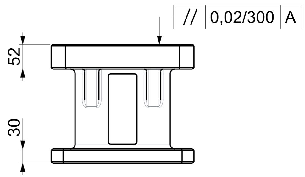
RISER TABLE - GIRDS HOLE Art.No. FG/WH/RISTL/RTG16NP003 Model.No.RTG/RT/600300/250-16
