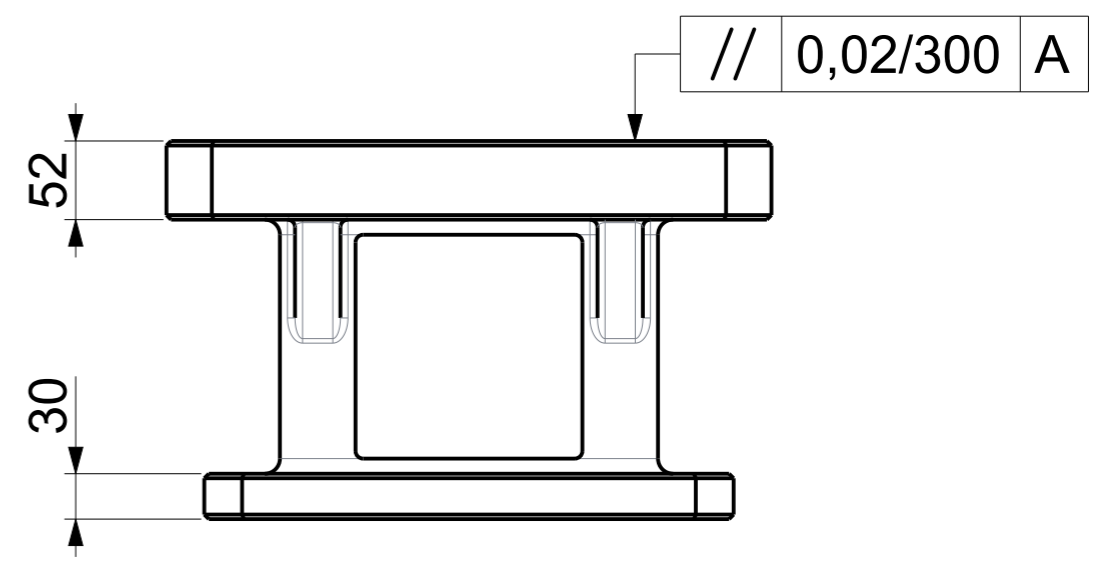
RISER TABLE - GIRD HOLE Art.No. FG/WH/RISTL/RTG16NP001 Model.No. RTG/SQ/400400/250-16
