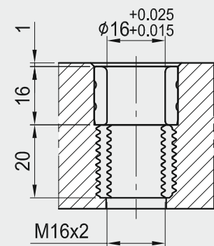
ø16 MTP hole
